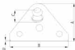
Fixing bracket 固定座
