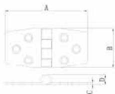
Door hinge 冲压合页
